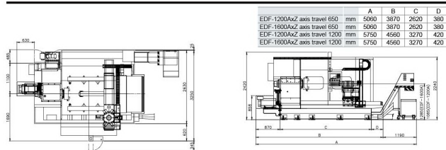
DIMENSIONS
