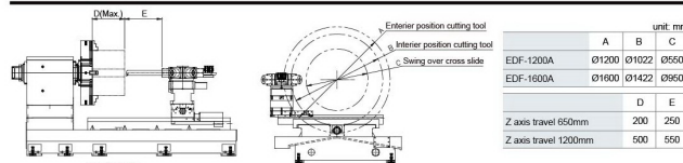
DIMENSIONS
