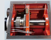
■ Headstock / 3-Step Hyd. Speed Shifting 主軸箱 / 三段油壓變速
