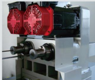
主軸頭: 2軸 / 4軸 Headstock: 2-axis / 4-axis
